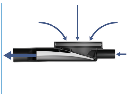
2 Når vannet renner inn i sluket åpnes membranvannlåsen og vannet renner
